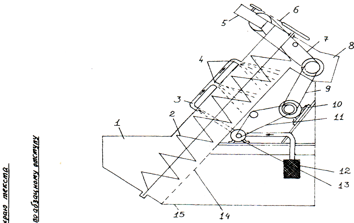
Рисунок 3.1 - Технологическая схема измельчителя ИКС-5М: 1- загрузочный бункер; 2 - шнек; 3 - напорная труба; 4 - патрубки с распределителями; 5 - редуктор; 6 – цепная передача; 7, 9, 11- клиноремённые передачи; 8 измельчающий аппарат; 10 - электродвигатель; 12 - фильтр; 13 - насос; 14 - сетка; 15 – ванна.
