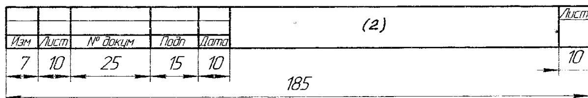
Рисунок 3 – Форма 2а основной надписи
