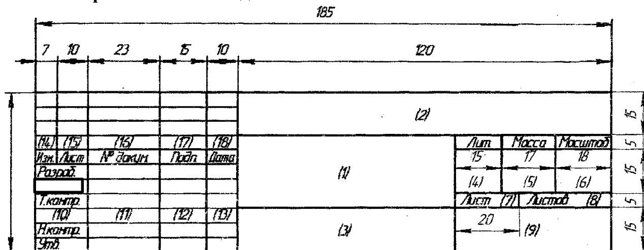
Рисунок 1 – Форма 1 основной надписи
