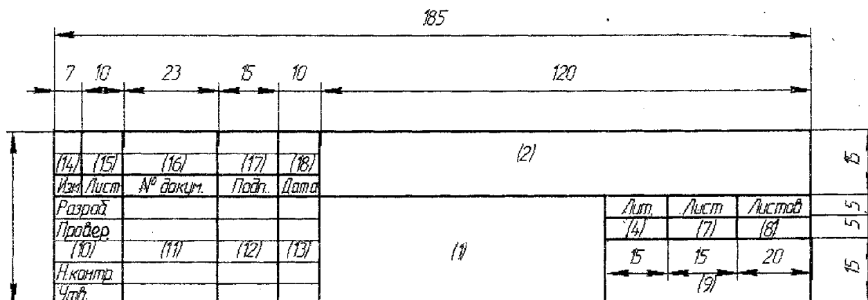
Рисунок 2 – Форма 2 основной надписи
