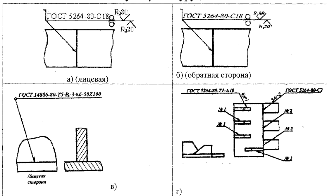
Рисунок 5 – Примеры обозначения сварных швов
