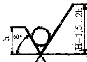
Рисунок 4 – Знаки обозначения шероховатости поверхности
